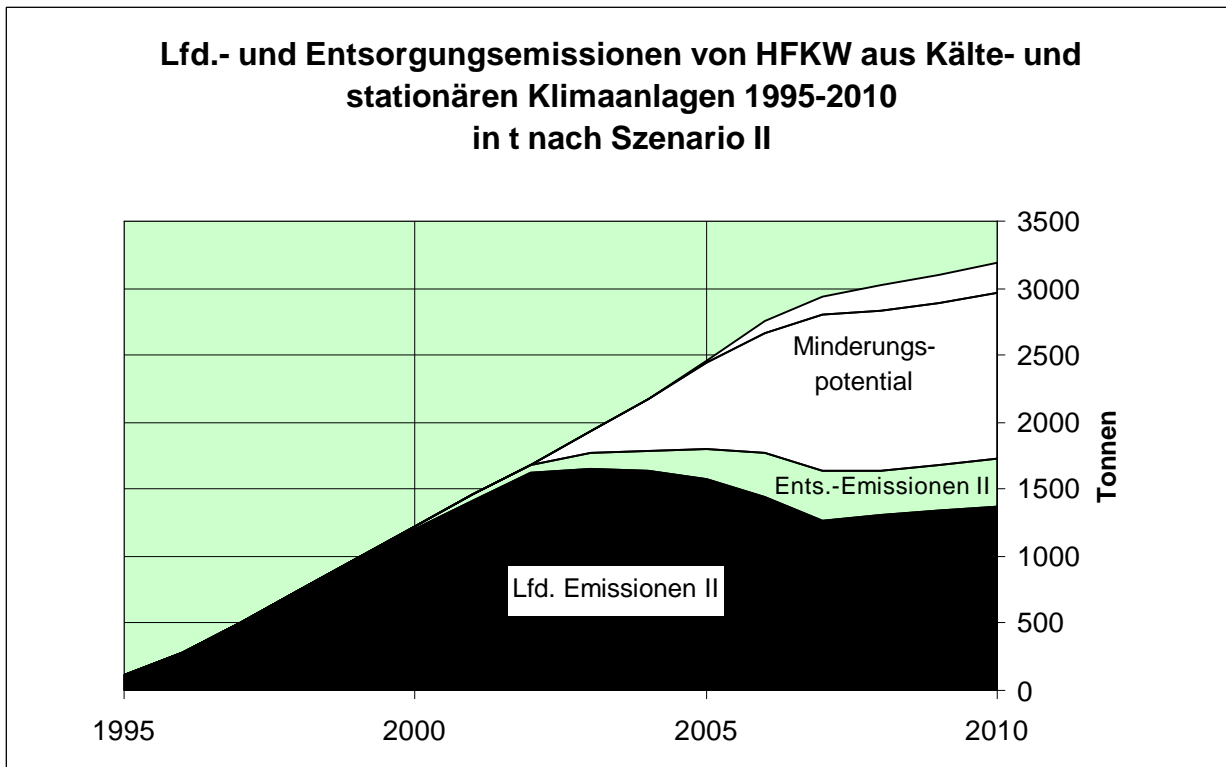
Diagramm 5: Lfd. und Entsorgungsemissionen von HFKW aus Kälte- und stationären Klimaanlage 1995-2010 in t - Szenario I u. II. Statt wie im Szenario I (alle Flächen zusammen) steigen die Emissionen nach 2003 nicht mehr. Die Summe aus Lfd. und Entsorgungsemissionen (dunkle Flächen) bleibt bis 2010 auf viel niedrigerem Niveau relativ konstant.
