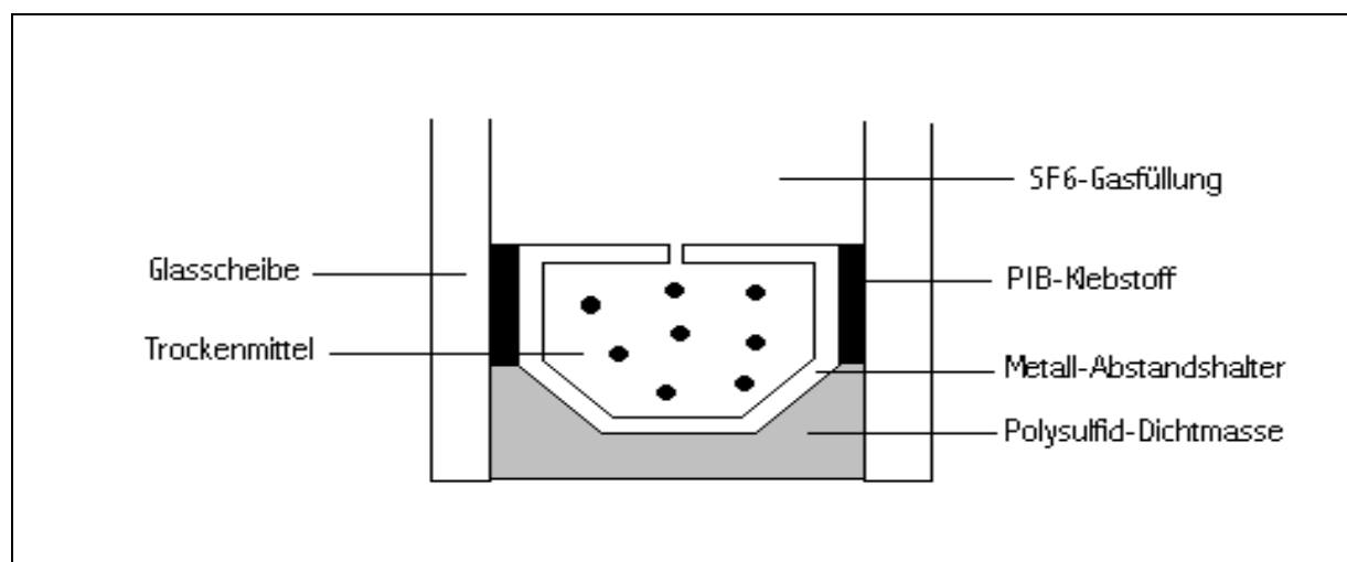
Abb. 2: Randverbund von Mehrscheiben-Isolierglas mit \text{SF}_6 -Füllung zum erhöhten Schallschutz. Der metallische Abstandshalter rund um die Kantenlänge der Scheiben ist mit einer Polysulfid-Masse gegen Diffusionen nach innen und außen abgedichtet. Das Trockenmittel saugt eindiffundierte Luftfeuchte 20 bis 30 Jahre lang auf. (Zeichnung nach Holler 1995, 69.)
