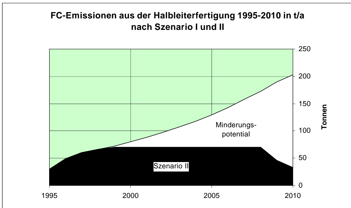
Diagramm 39: FC-Emissionen aus der Halbleiterfertigung 1995-2010 in t/a nach Szenario I und II. Werden entsprechend den Annahmen des Minderungsszenarios ab 2000 hocheffektive Plasmaverfahren eingesetzt, steigen im Unterschied zu Szenario I die Emissionen nicht mehr an, sondern sinken ab 2009 (Altanlagenersatz) sogar auf das Ausgangsniveau von 1995.
