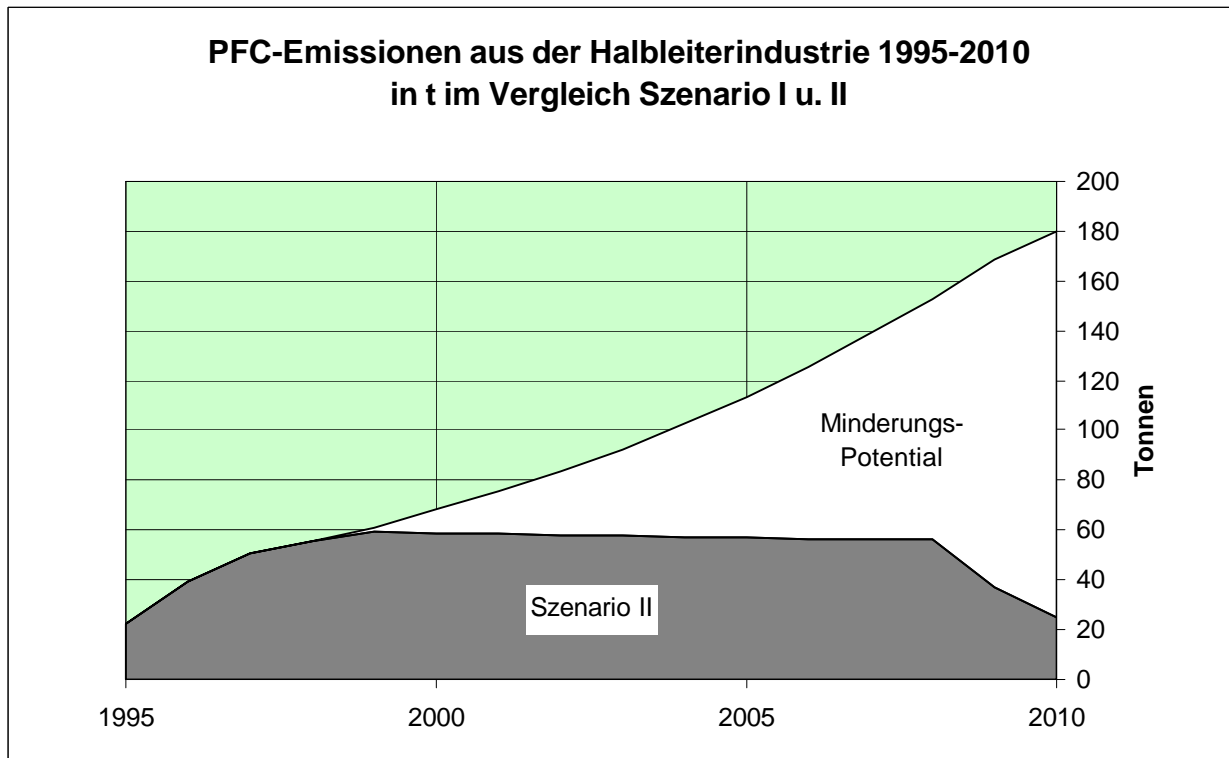
Diagramm 37: PFC-Emissionen aus der Halbleiterindustrie 1995-2010 in t im Vergleich Szenario I u. II. Im Unterschied zum BaU-Szenario, wo die Emissionen bis auf 181 t (2010) ansteigen, bleiben diese im Minderungsszenario ab 2000 konstant und sinken ab 2009. Aus der Differenz entsteht im Jahr 2010 ein Minderungspotential (weiße Fläche) von 156 t.
