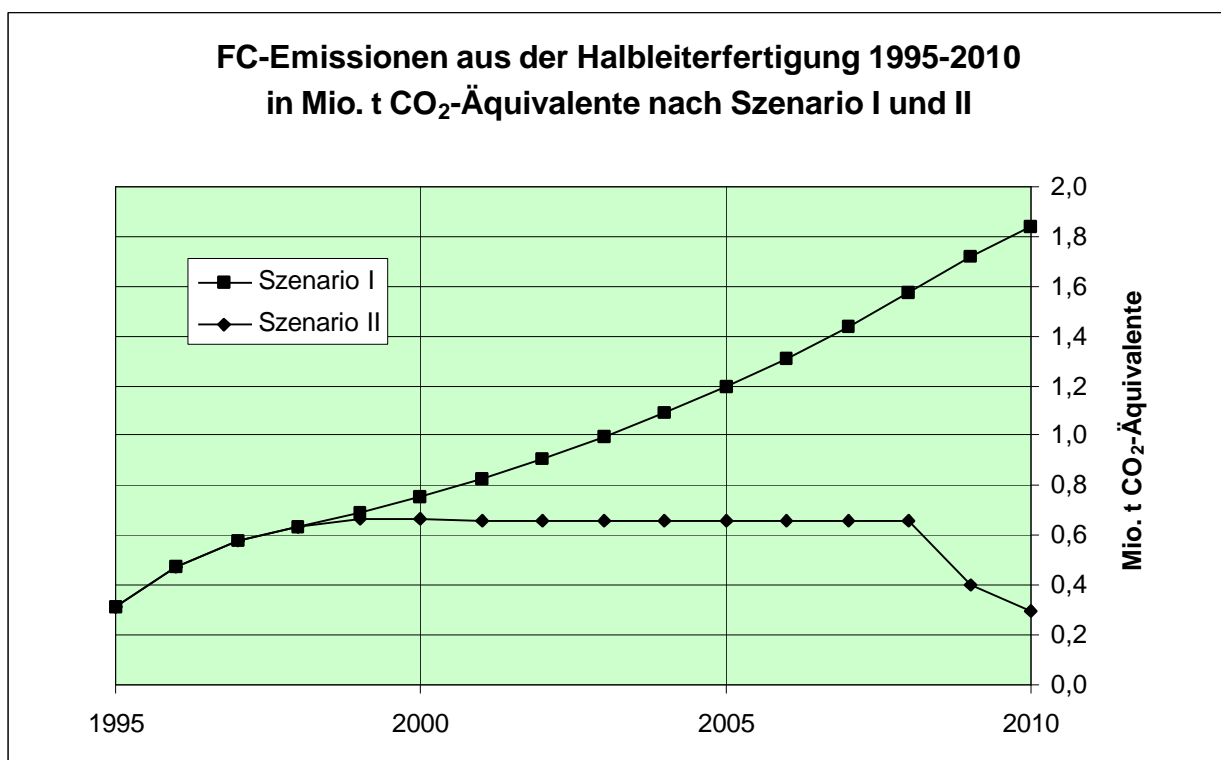
Diagramm 40: FC-Emissionen aus der Halbleiterfertigung 1995-2010 in Mio. t CO 2 -Äquivalente nach Szenario I und II. Nach BaU-Szenario I steigen die Emissionen bis 2010 auf über 1,8 Mio. t CO 2 -Äquivalente an. Unter den Bedingungen des Minderungsszenarios dagegen bleiben sie ab 2000 konstant und sinken bis 2010 auf 0,295 Mio. t - unter den Ausgangswert von 1995.
