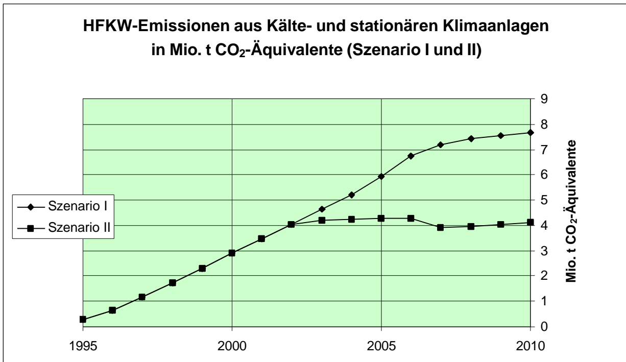
Diagramm 6: HFKW-Emissionen aus Kälte- und stationären Klimaanlage in Mio. t CO 2 -Äquivalente (Szenario I und II). Ab 2003 steigt der Beitrag zum Treibhauseffekt in Szenario II nicht mehr weiter an - wie das in Szenario I der Fall ist.
